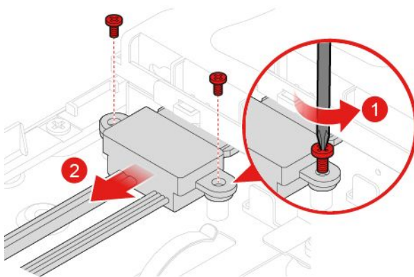
图 25. 卸下光盘驱动器和存储驱动器线缆
