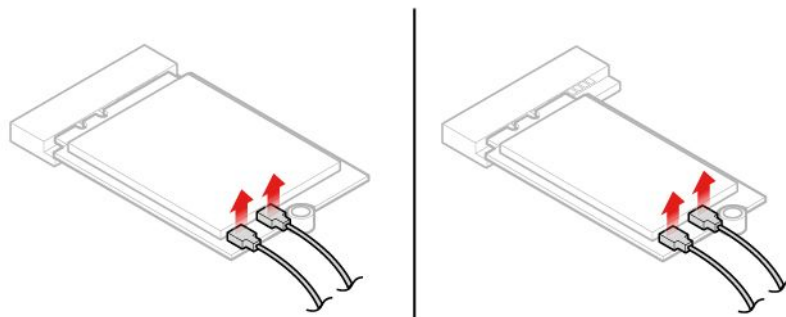
图 52. 拔下 Wi-Fi 天线线缆
