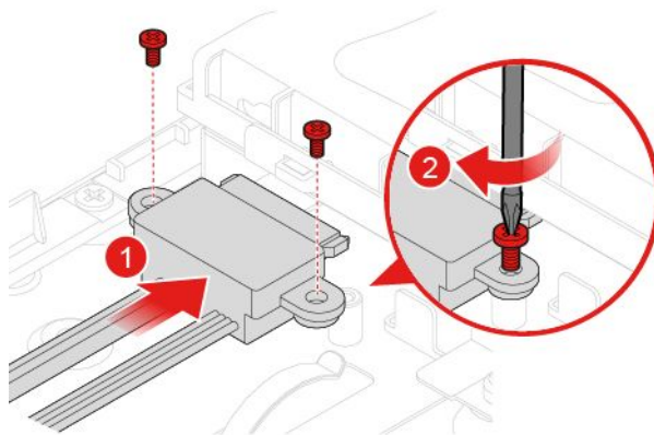
图 26. 安装光盘驱动器和存储驱动器线缆
