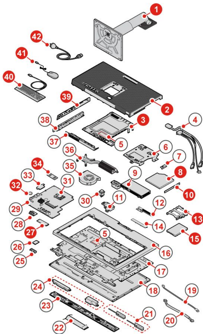
图 9. 确定 FRU 的位置 (包括 CRU)
