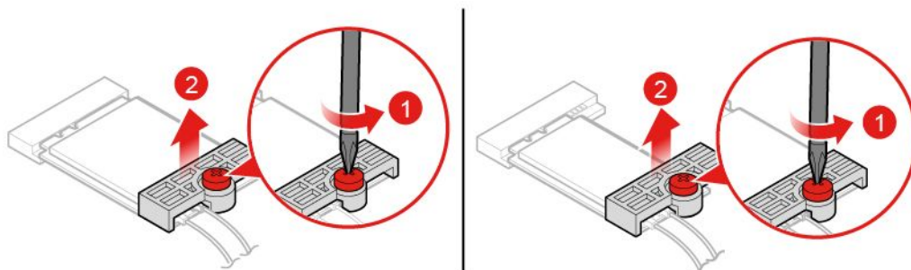
图 51. 卸下 Wi-Fi 卡蔽罩
