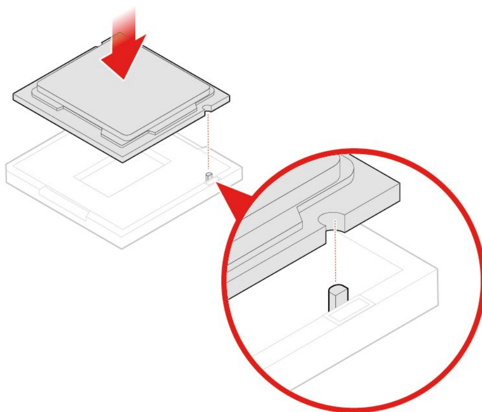
图 48. 安装微处理器
