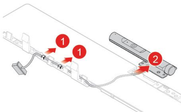
图 80. 拔下并移除集成摄像头和麦克风模块线缆
