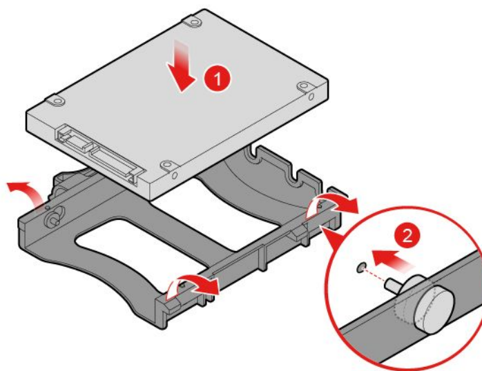
图 15. 将存储驱动器装入支架中
