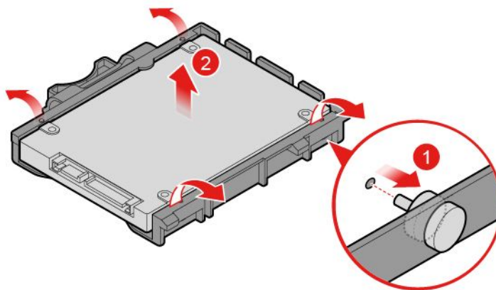
图 14. 从支架上卸下存储驱动器
