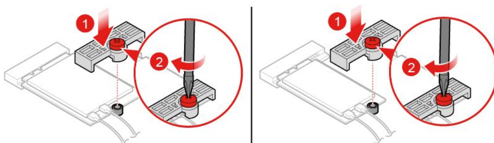
图 56. 安装 Wi-Fi 卡蔽罩
