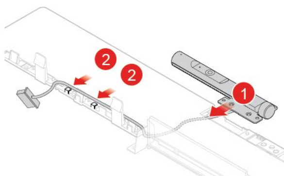
图 81. 安装并连接集成摄像头和麦克风模块线缆
