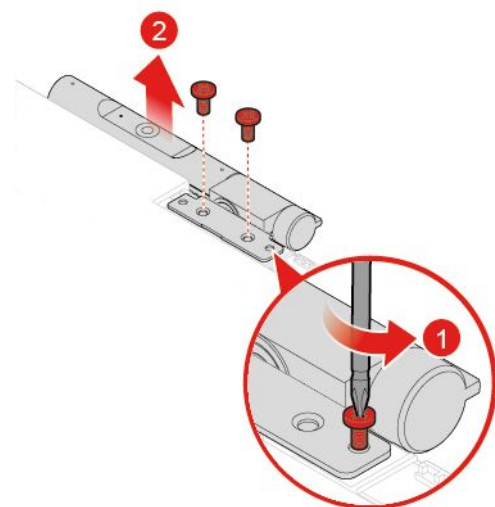
图 79. 从背框上卸下集成摄像头和麦克风模块
